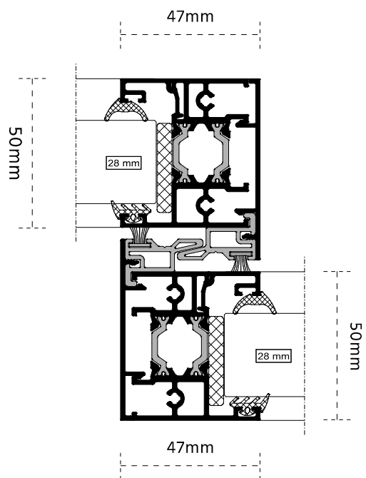
Slimline interlock
